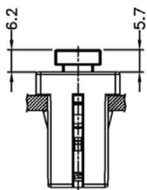
下壓時最大行程 (Pressed fastening)
