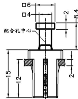
未扣合視圖(Unfastening)
