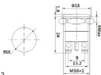
GQ-16F-2 3A 250VAC ; 2A 36VDC
