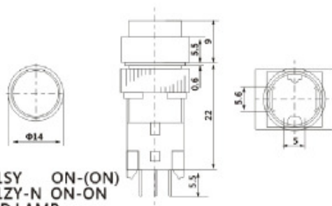
KD19-3 15A 250VAC
