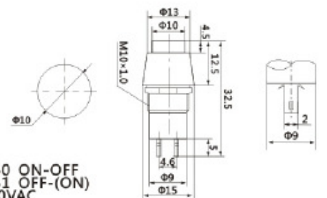
CS-450 ON-OFF CS-451 OFF-(ON) 1A 250VAC
