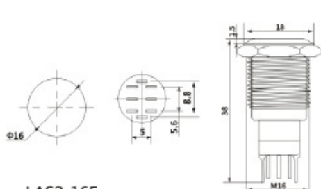
LAS2-16F 3A 250VAC ; 2A 36VDC
