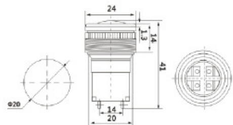
AN24-Z ON-(ON) SPDT 4PIN AN24-2H OFF-(ON) DPST 4PIN 6A 250VAC; 10A 125VAC
