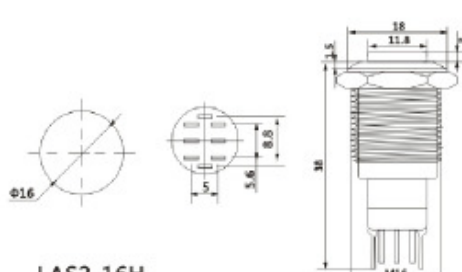
LAS2-16H 3A 250VAC ; 2A 36VDC
