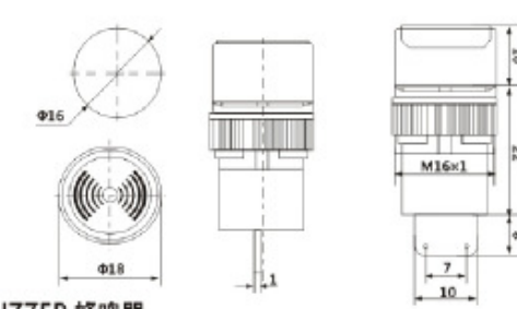
A16 BUZZER 蜂鸣器
